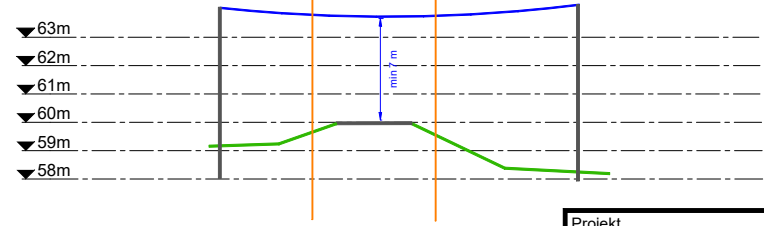
RV-1: õhuliini ristumine 69 Võru-Kuigatsi-Tõrva teega km.61,85
